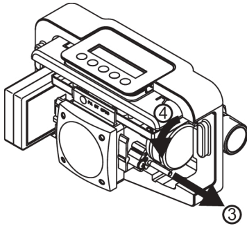
Abb. 8: Roten Arretierstift entfernen und Motor drehen
